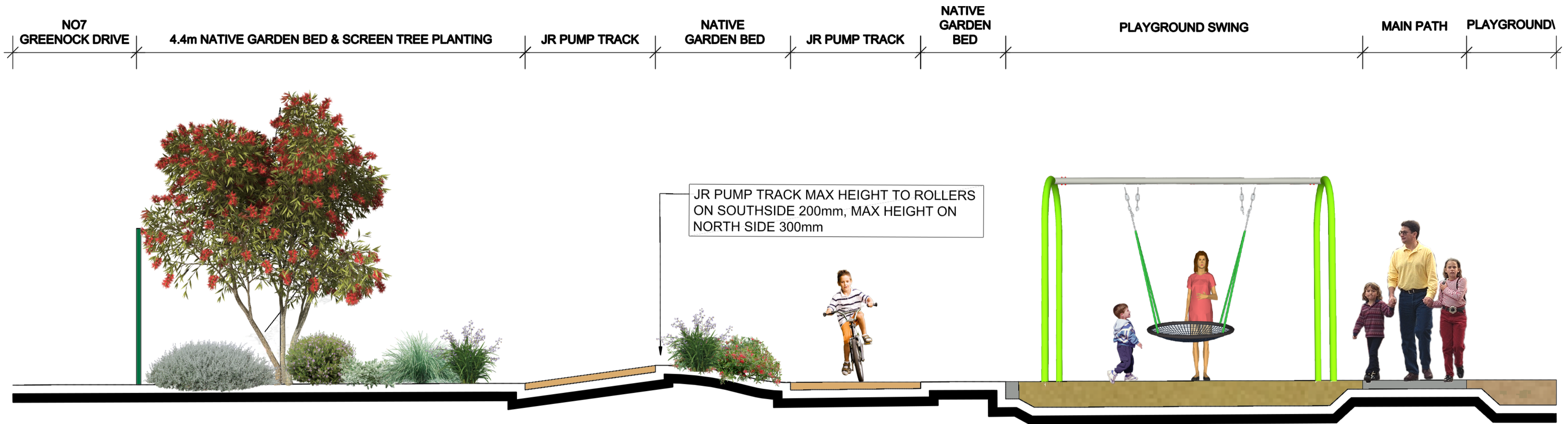
SECTION A-A
